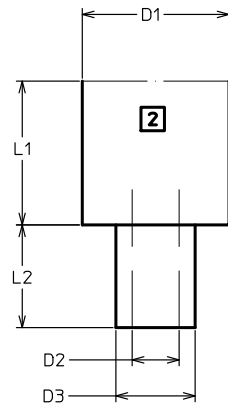
Mandrino DIN 55058 DIN 55058 Spindle
