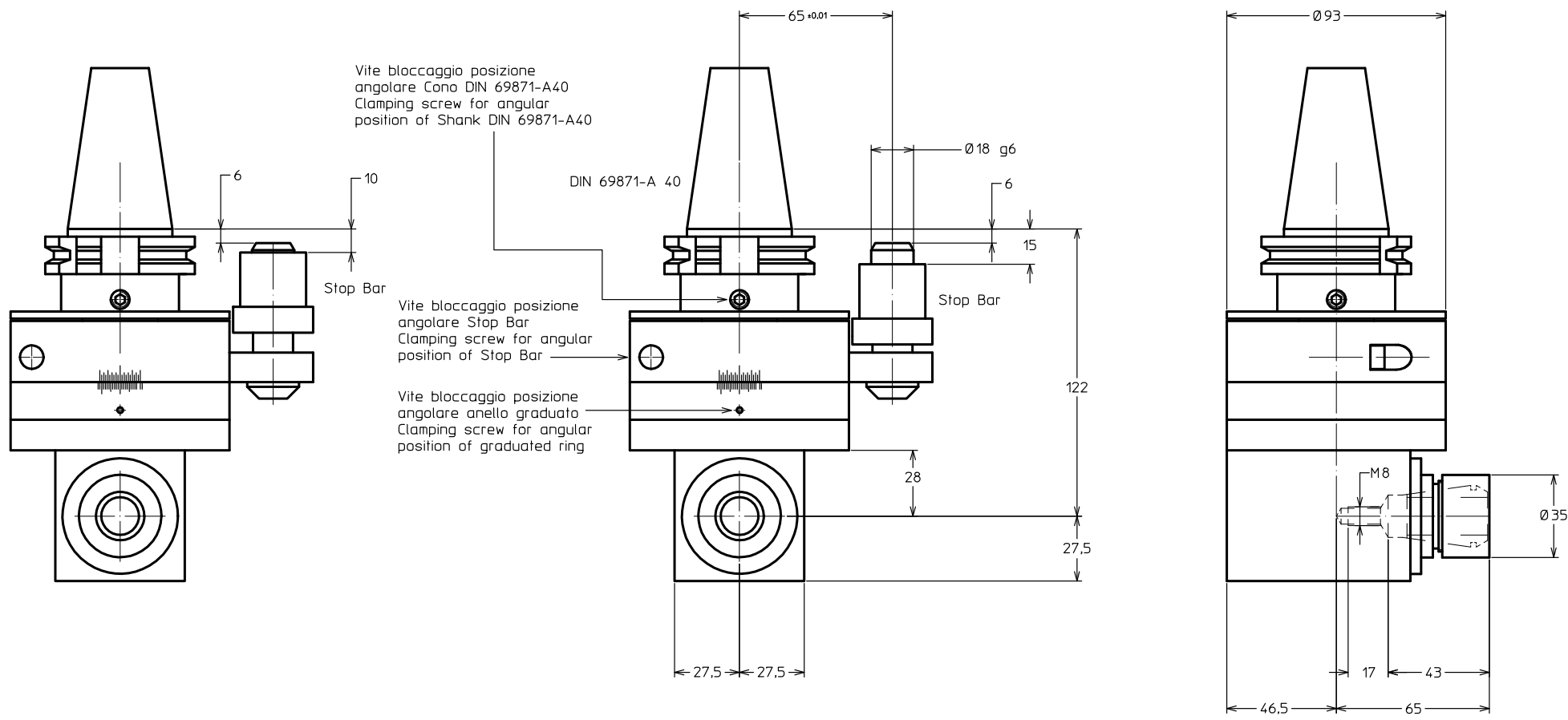
Mandrino per pinza ER 25 Spindle for collet ER 25
