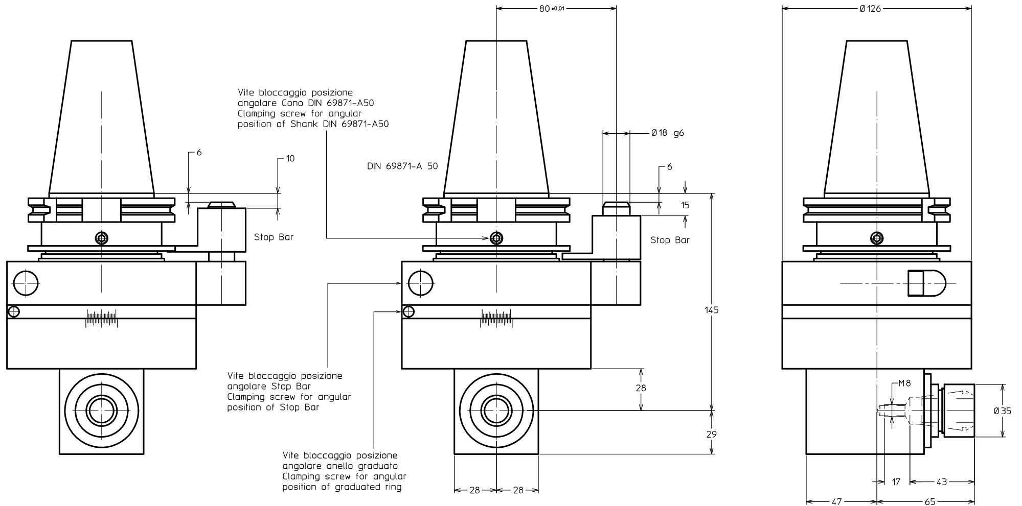
Mandrino per pinza ER 25 Spindle for collet ER 25
