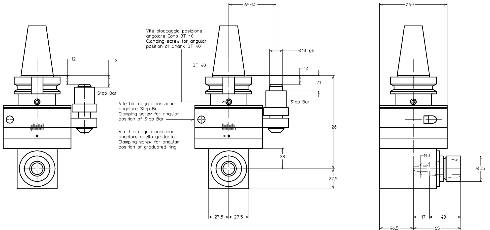
Mandrino per pinza ER 25 Spindle for collet ER 25
