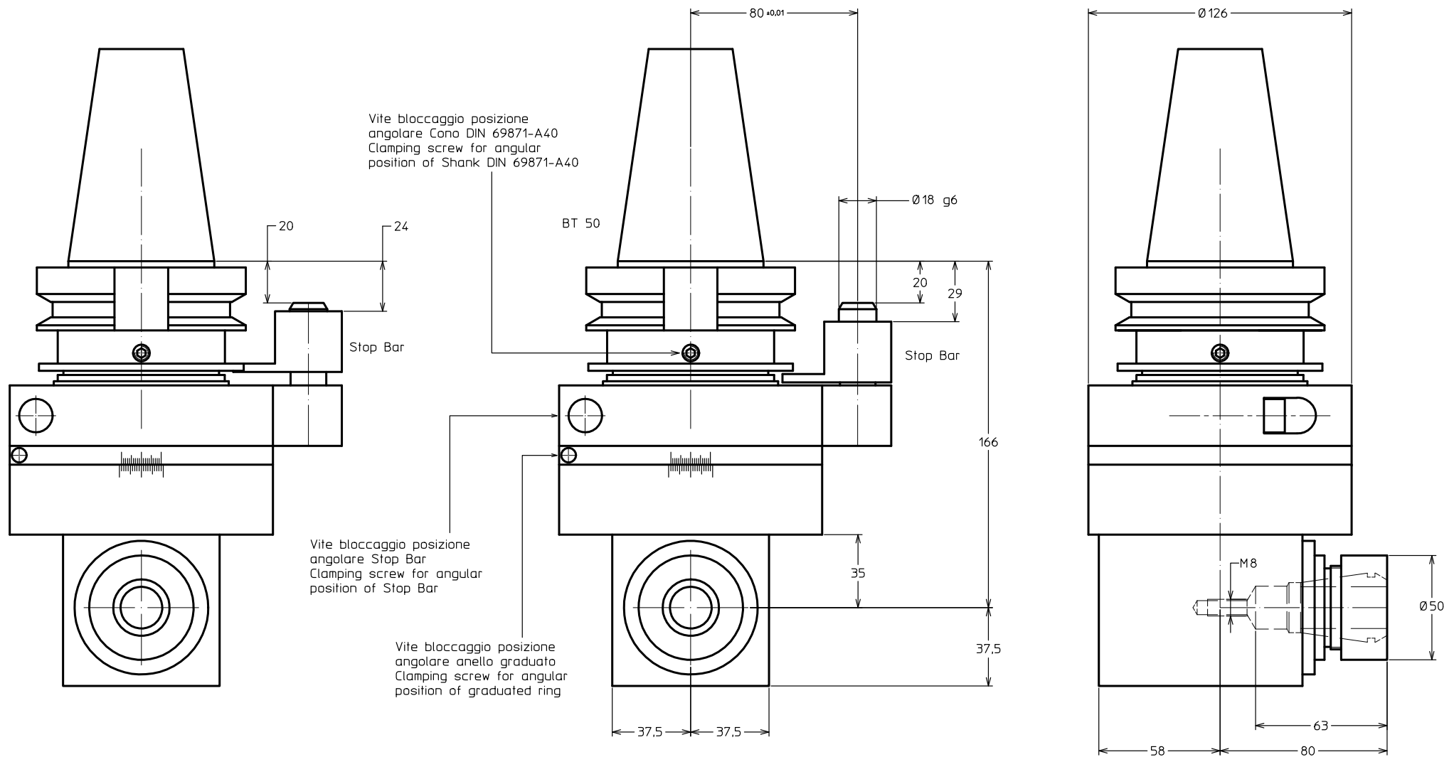
Mandrino per pinza ER 32 Spindle for collet ER 32
