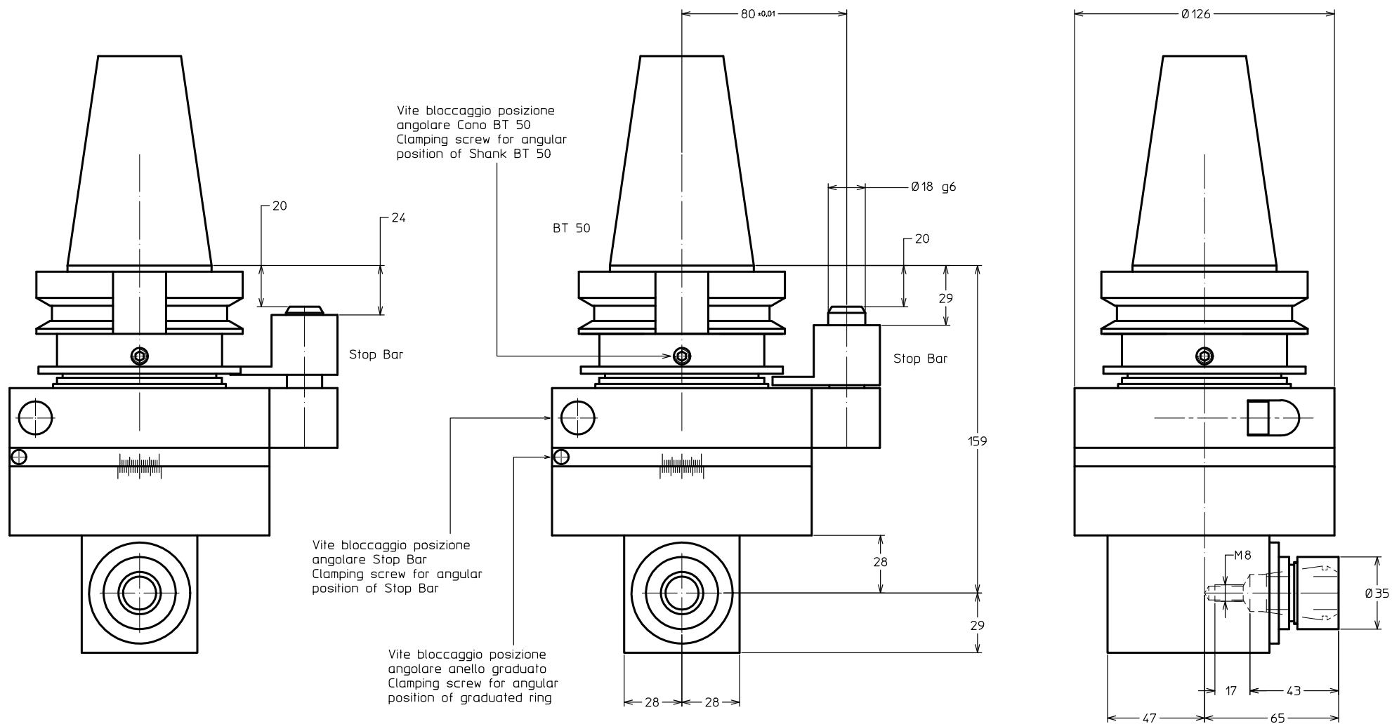
Mandrino per pinza ER 25 Spindle for collet ER 25
