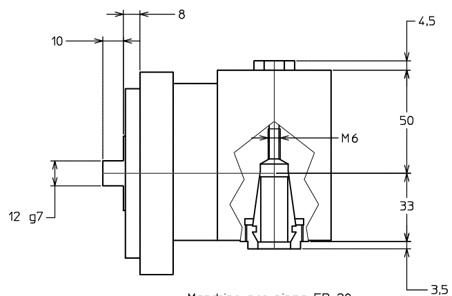
Mandrino per pinza ER 20 Spindle for collet ER 20
