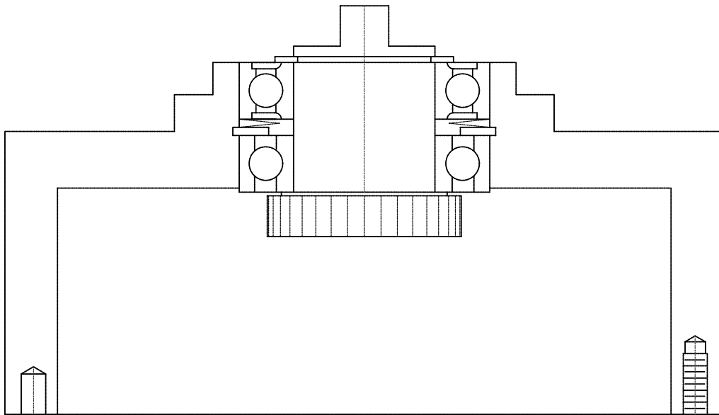
GR. PRESA DI FORZA MAIN DRIVE UNIT 117031-100
