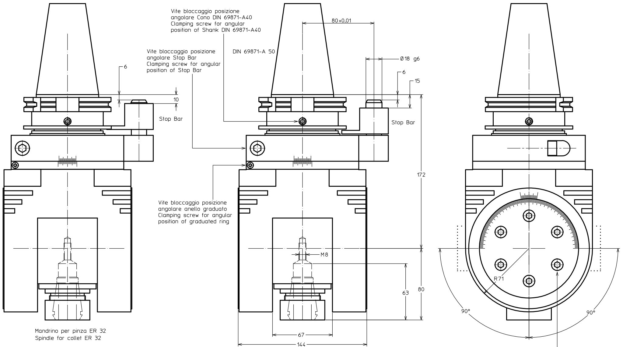
Vite bloccaggio posizione angolare mandrino Clamping screw for angular position of spindle
