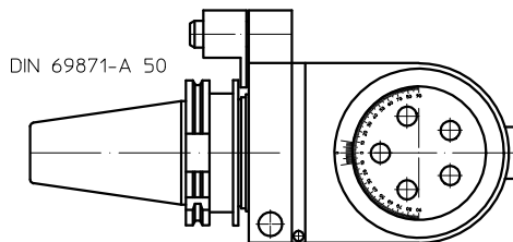
Tipo / Type T25CN-50 Codice / Code 124907.100 Mandrino / Spindle ER 25
