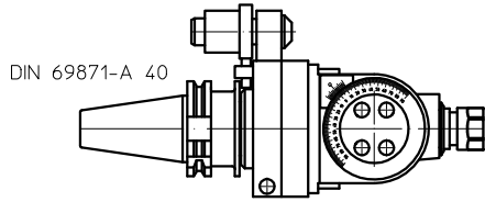
Tipo / Type T16CN-40 Codice / Code 124920-100 Mandrino / Spindle ER 16
