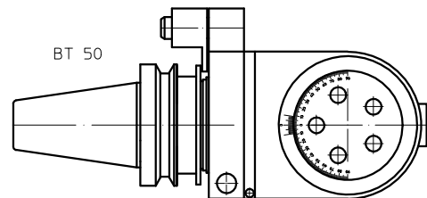
Tipo / Type T25CN-BT50 Codice / Code 124913.100 Mandrino / Spindle ER 25
