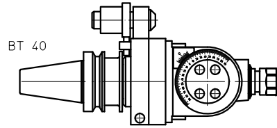
Tipo / Type T16CN-BT40 Codice / Code 124921-100 Mandrino / Spindle ER 16
