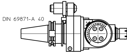
Tipo / Type T20CN-40 Codice / Code 124936-100 Mandrino / Spindle ER 20
