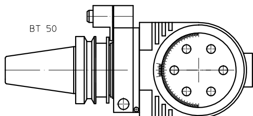
Tipo / Type T32CN-BT50 Codice / Code 124914.100 Mandrino / Spindle ER 32
