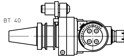
Tipo / Type T20CN-BT40 Codice / Code 124937-100 Mandrino / Spindle ER 20
