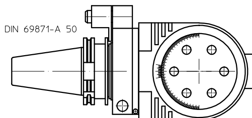
Tipo / Type T32CN-50 Codice / Code 124910.100 Mandrino / Spindle ER 32
